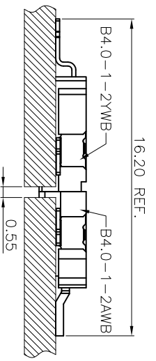
产品互配视图
